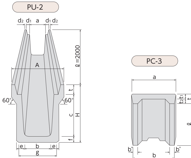
本体 PU-2 (歩道用) 寸法表
